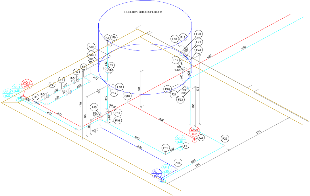
Detalhe Hidráulico-10 Escala 1:25
